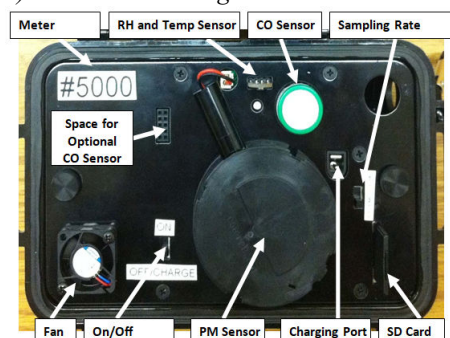
Fig. 16. IAP meter
